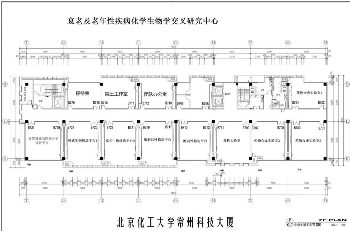
七层布局
