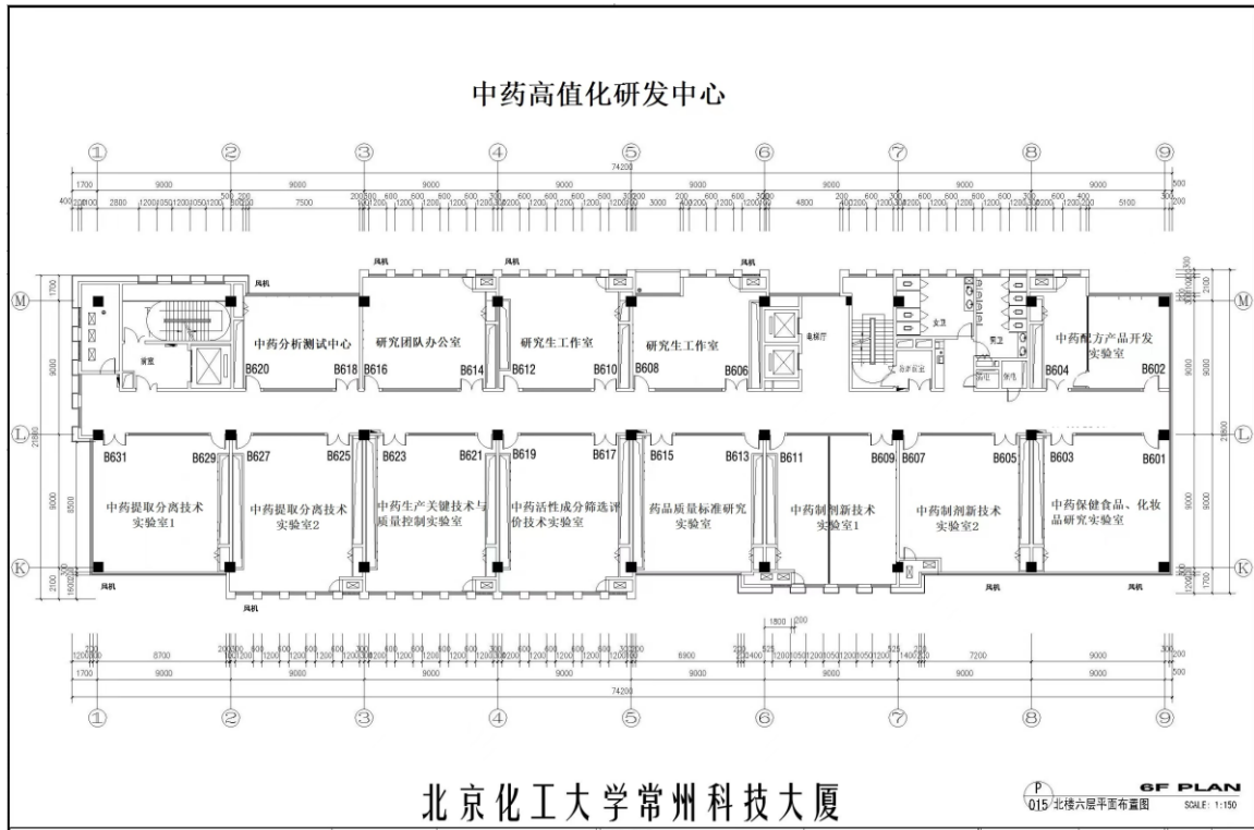
六层布局
